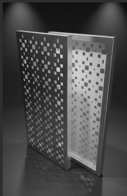
JÚPITER IO
