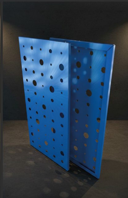
SATURNO
