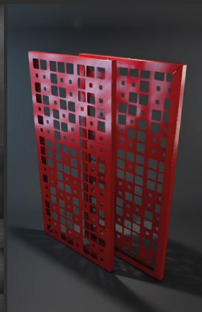
JÚPITER
