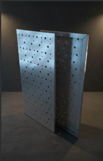
PLUTÓN
